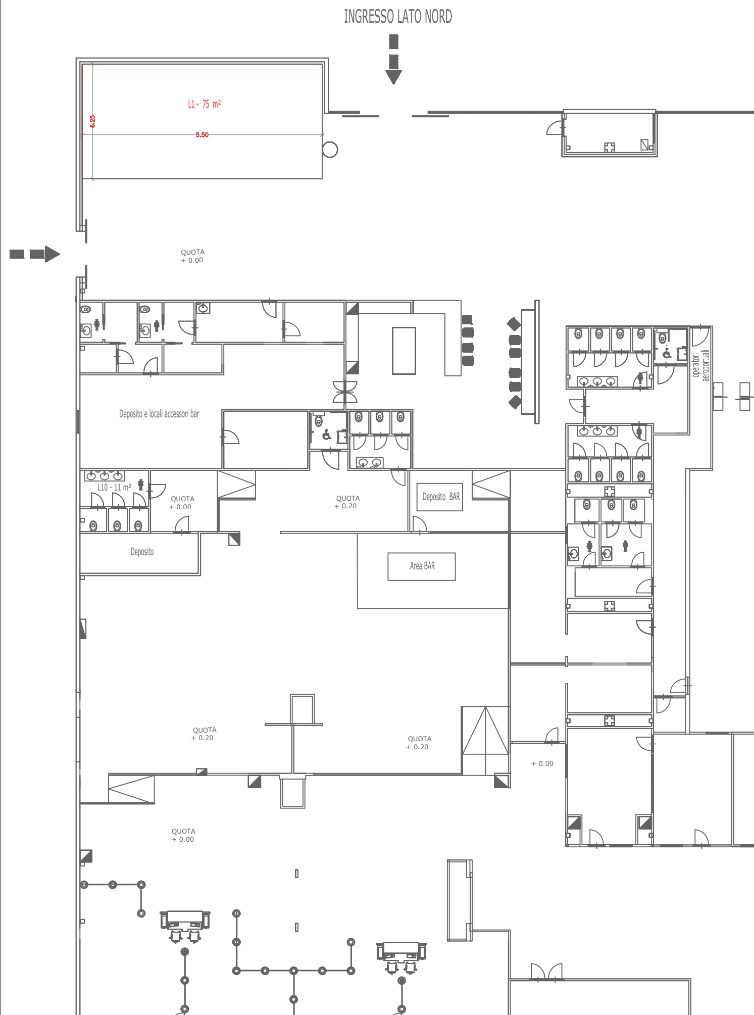
PLANIMETRIA DI DETTAGLIO Scala 1:200
